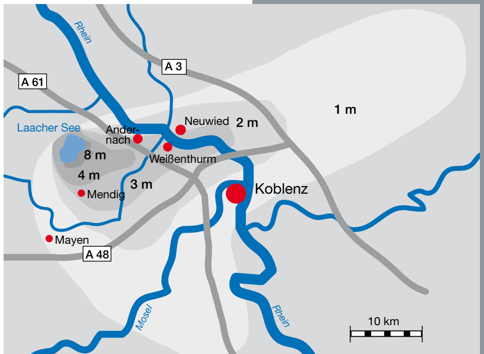
Mächtigkeitsverteilung der Bimsablagerungen des Laacher See Vulkans im Neuwieder Becken.
